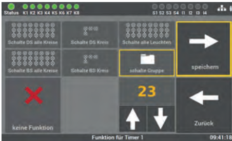
Abb. 106: Maske „Zeitschaltuhren – Aktionsauswahl“
