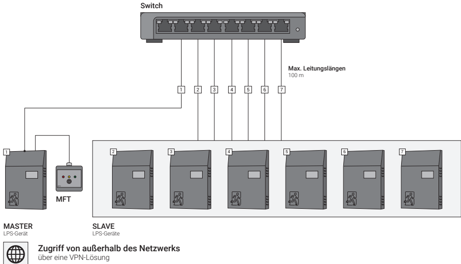
Abb. 158: Übersicht für den Einsatz von mehreren LPS-Geräten (ohne DHCP-Server)
