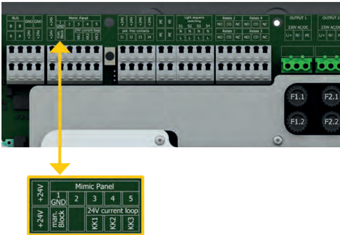
Abb. 25: Notlichtblockierung
