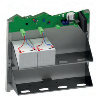
Abb. 10: Batterieaufbau 12 Ah
