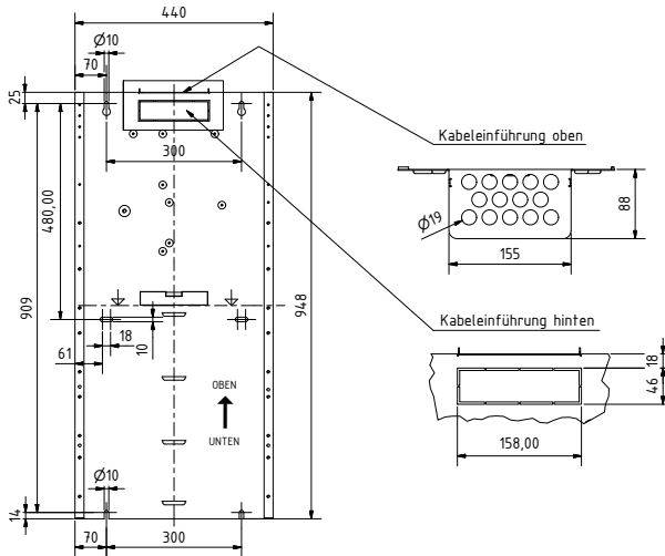
Abb. 8: Ansicht LPS-Montageplatte von vorne (Abmessungen ohne Abdeckung)
