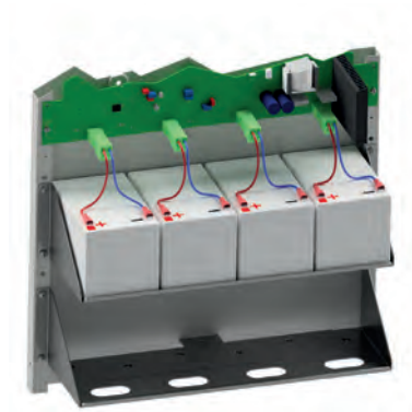
Abb. 11: Batterieaufbau 24 Ah
