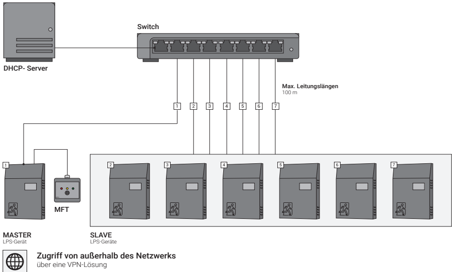
Übersicht für den Einsatz von mehreren LPS-Geräten
