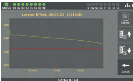
Abb. 69: Maske „Ergebnis letzter Betriebsdauertest“
