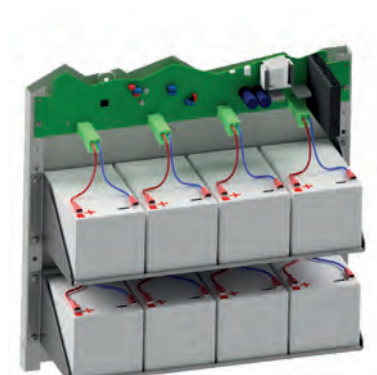
Abb. 13: Batterieaufbau 48 Ah
