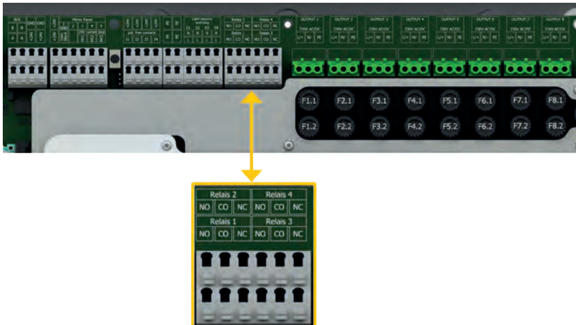
Abb. 24: Relaisausgänge
