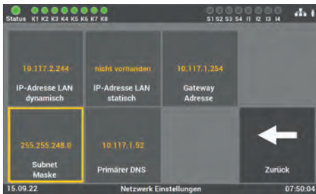
Abb. 137: Maske „Adresse Subnetz“
