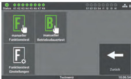
Abb. 76: Menüpunkt „Testmenü“
