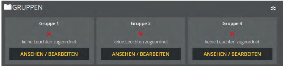
Abb. 191: Gruppen
