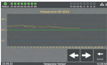
Abb. 70: Maske „Temperaturüberwachung“
