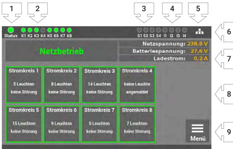
Abb. 52: Displaybedienung
