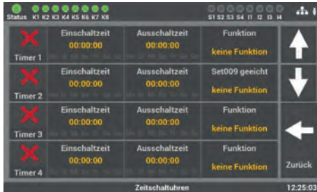
Abb. 103: Maske „Zeitschaltuhren“
