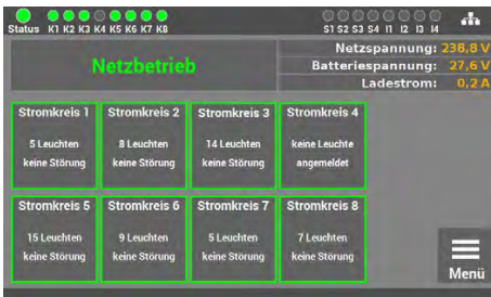
Abb. 49: Start-Maske (Einzelleuchtenüberwachung)
