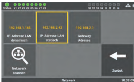
Abb. 133: IP-Adresse
