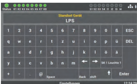
Abb. 102: Maske „Ortseingabe“
