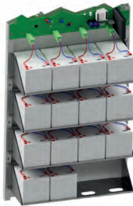
Abb. 16: Batterieaufbau 84 Ah
