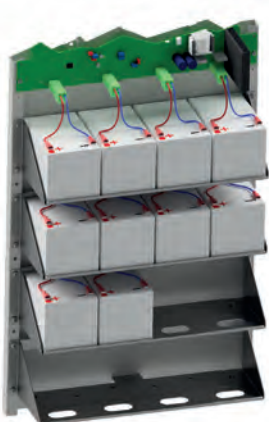
Abb. 14: Batterieaufbau 60 Ah
