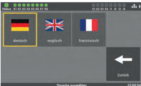
Abb. 150: Maske „Sprache“
