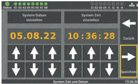
Abb. 125: Maske „Datum/Uhrzeit“
