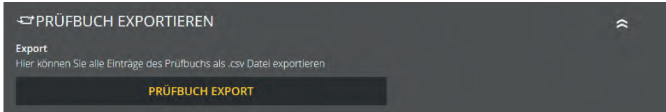
Abb. 184: Prüfbuch exportieren
