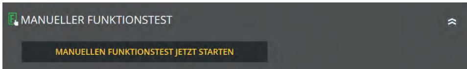
Abb. 185: manueller Funktionstest
