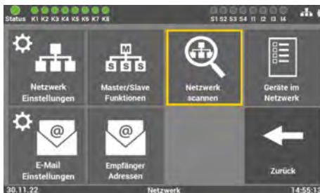
Abb. 141: Maske „Netzwerkscan“
