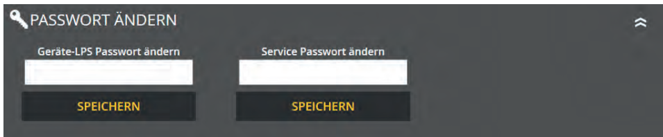
Abb. 200: Passwort ändern
