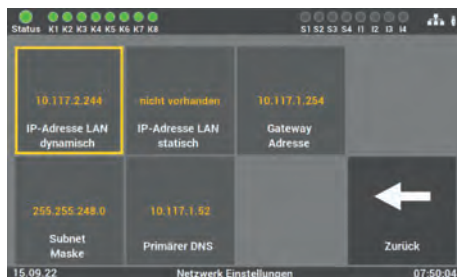
Abb. 132: DHCP-Adresse
