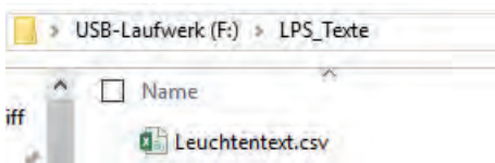
Abb. 100: Ordnerstruktur
