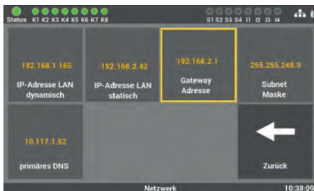
Abb. 135: Gateway-Adresse
